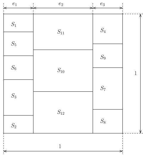
FIG. 1 – Partitionnement du carré unité en colonnes de rectangles.
